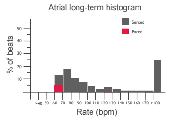
Arrhythmia
