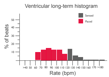
% biventricular pacing
